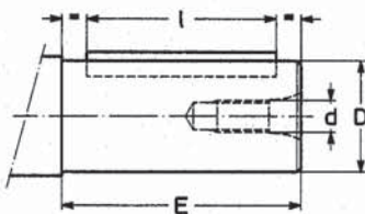
Estremità d'albero - Shaft end
