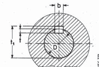
Albero lento cavo - Hollow low speed shaft
