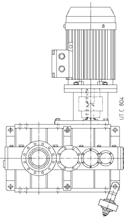
Sistema di reazione (cap. 15) semielastico ed economico: con bullone a molle a tazza, con bullone a molle a tazza con forcella.
