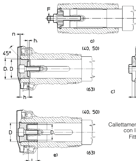
Fissaggio assiale Axial fastening
